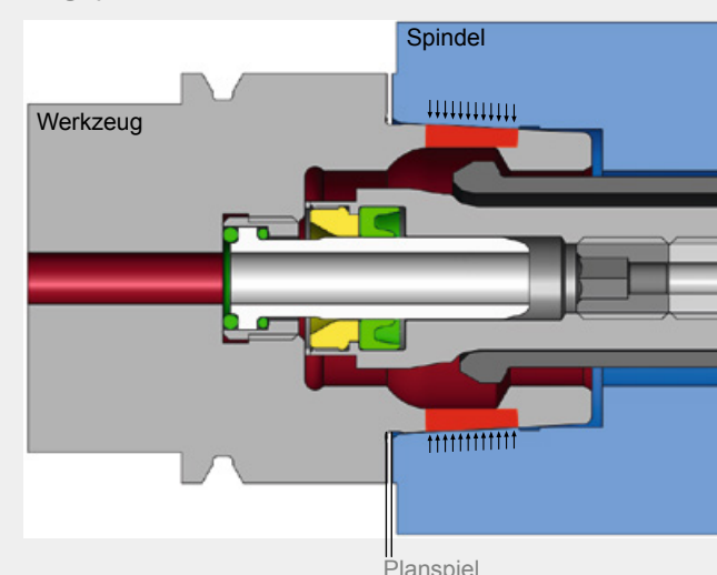
Fügeposition
